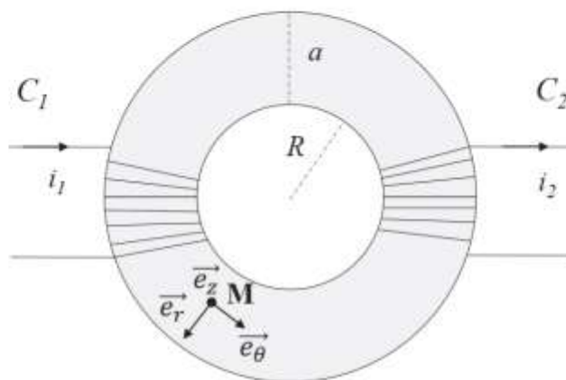
Figure 1 – Vue de dessus du transformateur
